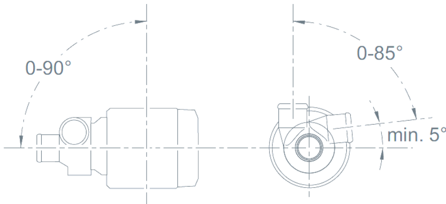
Målskisse AquaVent 6000SC ( U4856 )
