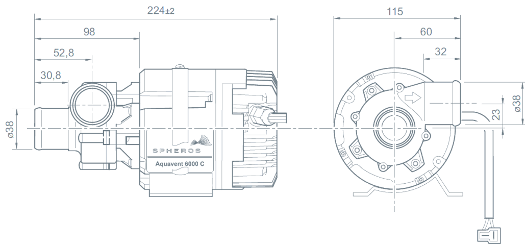
Målskisse AquaVent 6000C ( U4855 )
